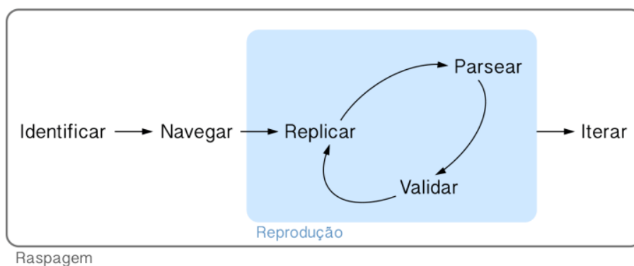
Figura 2.15: Ciclo da raspagem de dados. Fonte: curso de Web Scraping da Curso-R
